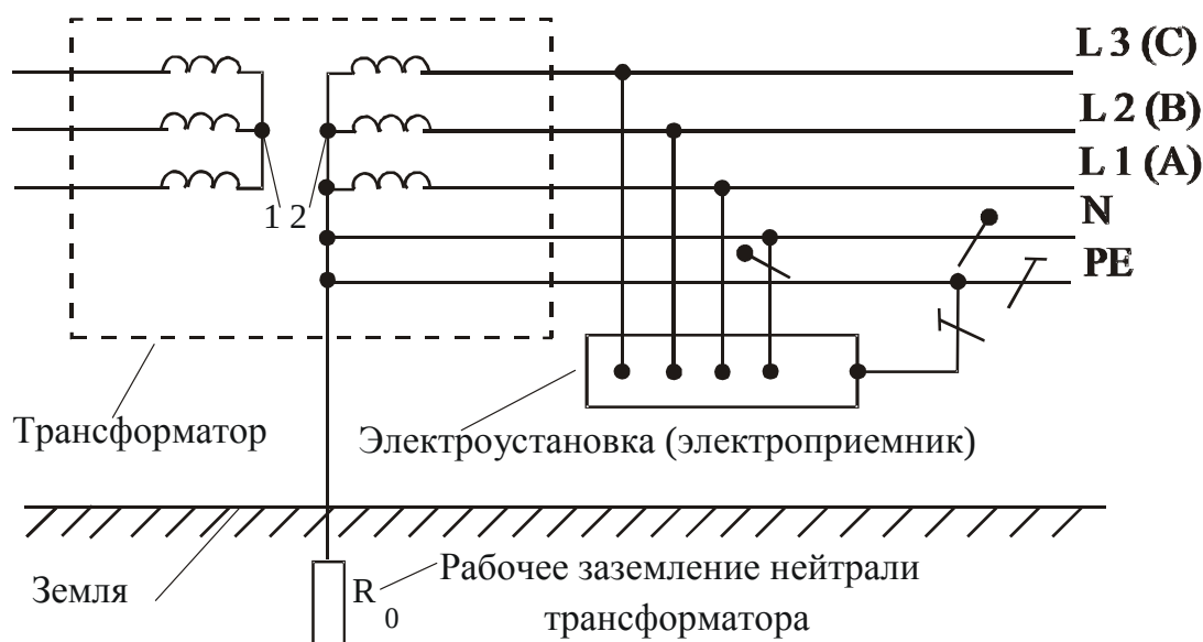
Рис. 6.4. Трехфазная сеть с подключенным к ней электроприемником
