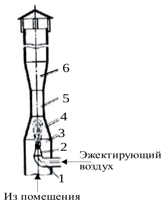
Рис. 4.4. Схема работы эжектора
