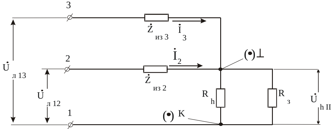
Рис. 6.12. Эквивалентная схема II варианта
