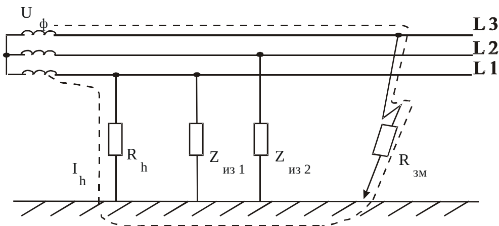
Рис. 6.6. Трехфазная сеть с изолированной нейтралью (IT) в аварийном режиме работы
