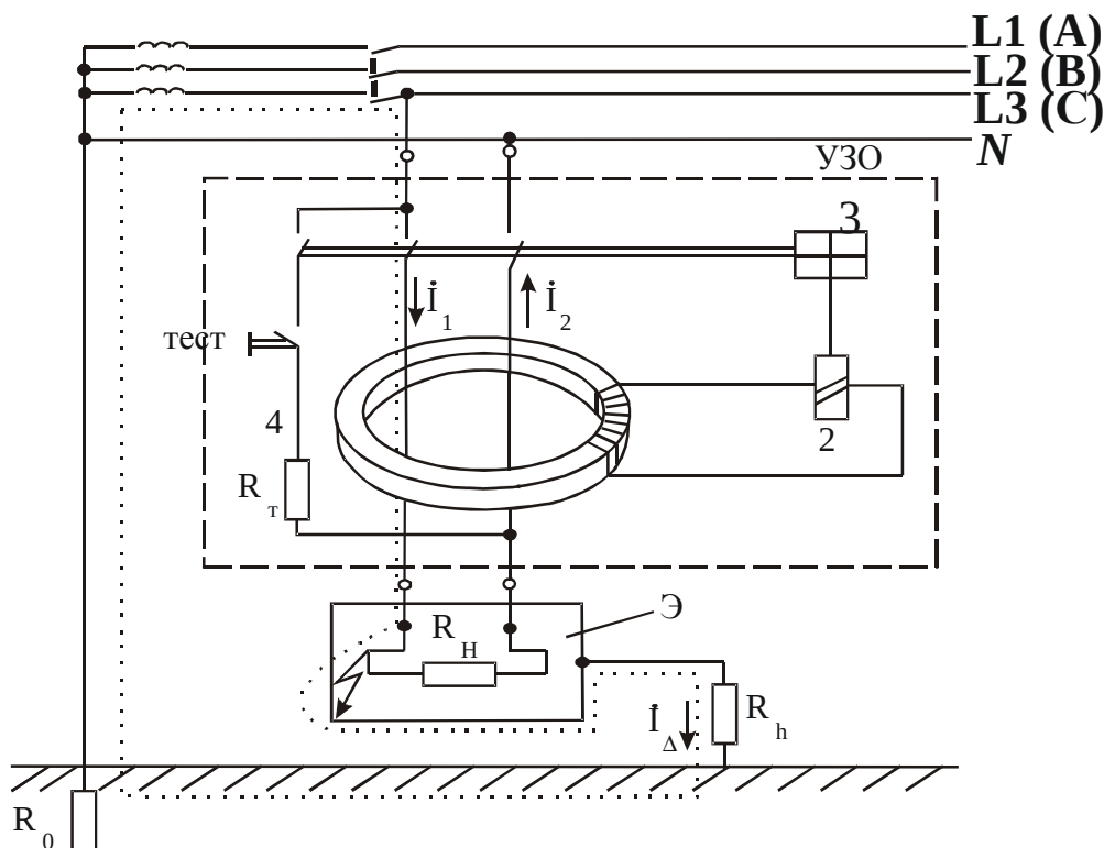
Рис. 6.18. УЗО, реагирующее на дифференциальный ток
