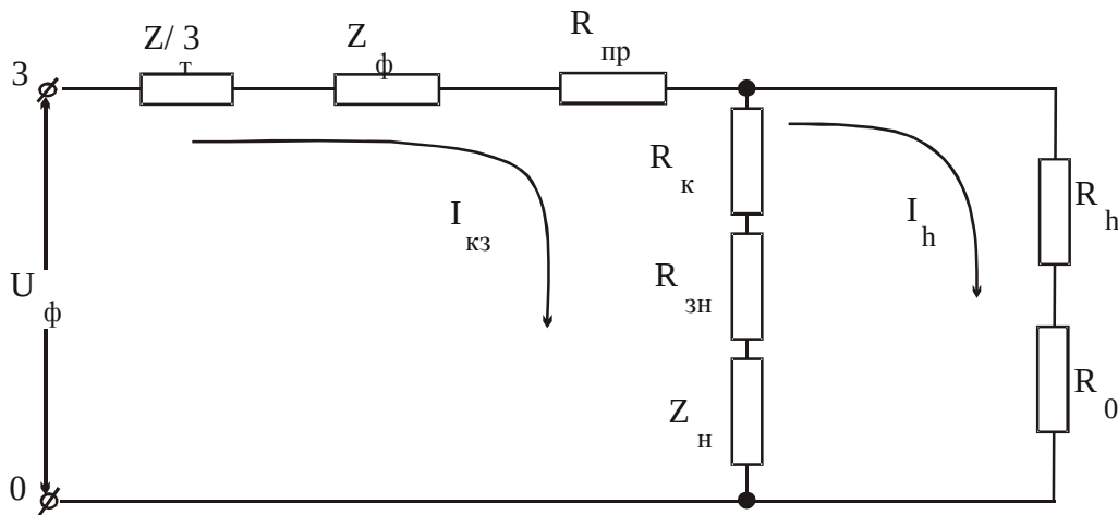
Рис. 6.14. Эквивалентная схема зануления при отсутствии повторного заземления нулевого провода R_n
