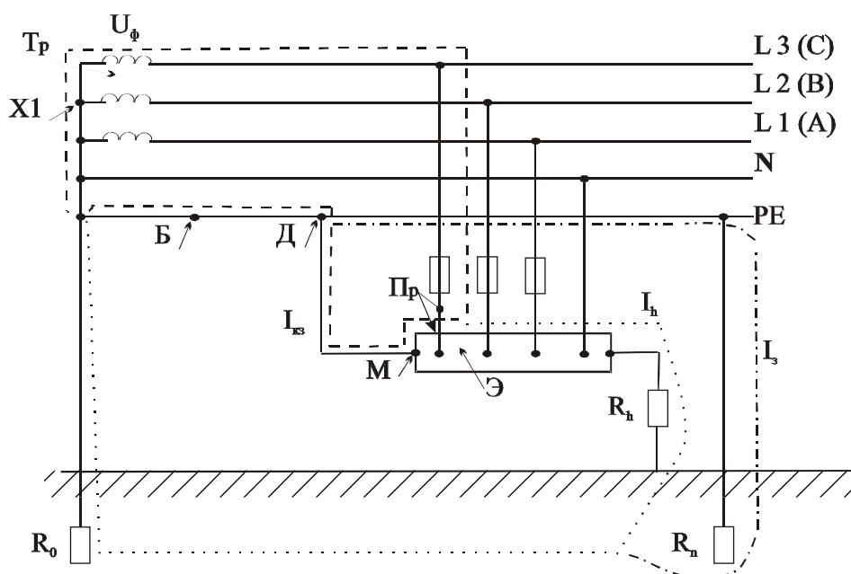
Рис. 6.13. Зануление и повторное заземление нулевого провода в трехфазной пятипроводной сети с глухозаземленной нейтралью напряжением до 1 кВ (система TN-S)
