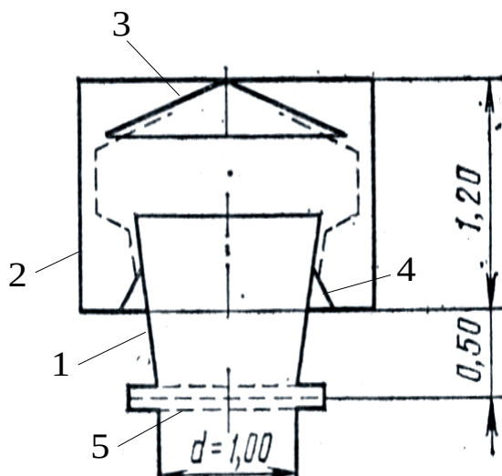
Рис. 4.3. Дефлектор ЦАГИ
