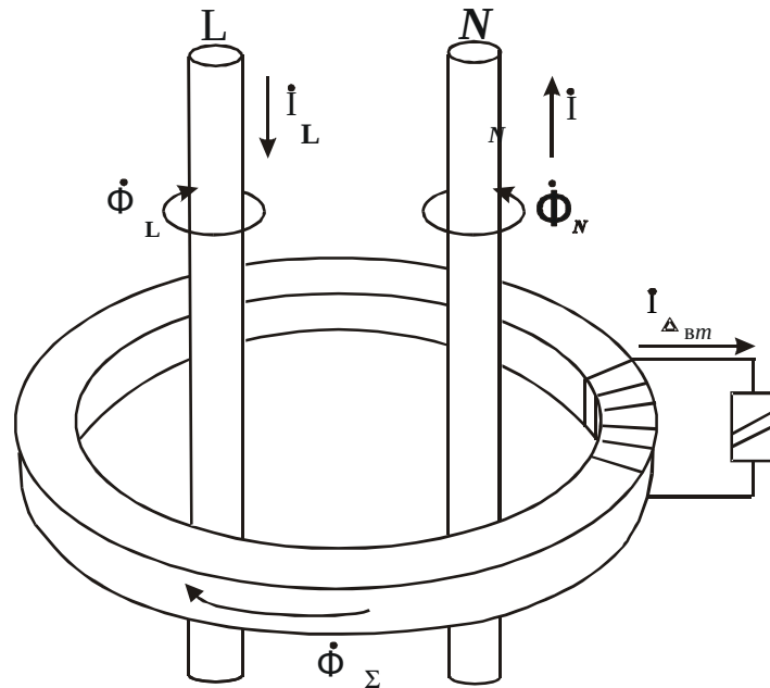
Рис. 6.17. Дифференциальный трансформатор тока
