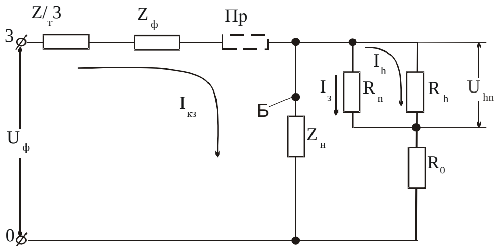
Рис. 6.16. Эквивалентная схема зануления при наличии повторного заземления нулевого провода R_n
