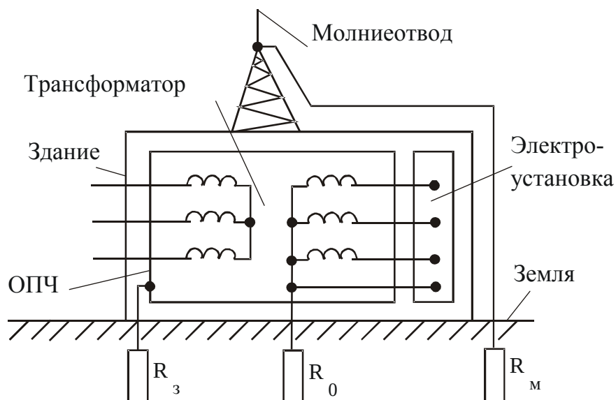
Рис. 6.9. Заземление: R_0 – рабочее; R_m – молниезащиты; R_z – защитное
