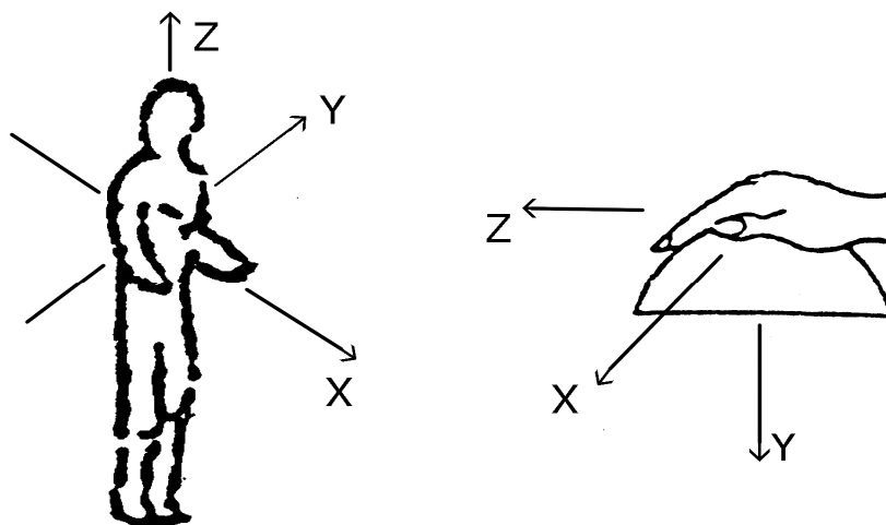
Рис. 4.1. Расположение осей системы координат для определения направления вибрации
