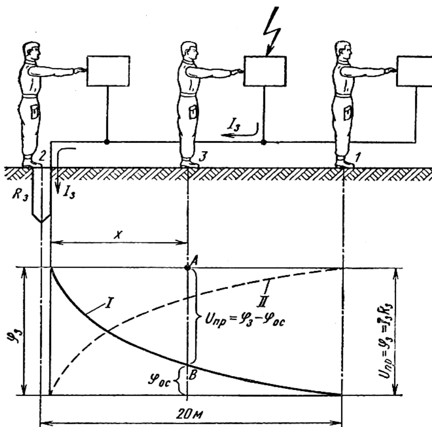
Рис. 6.2. Напряжение прикосновения при одиночном заземлителе: I – потенциальная кривая; II – кривая, характеризующая изменение напряжения прикосновения U_{пр} при изменении расстояния от заземлителя x
