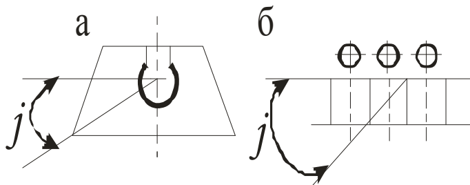
Рис. 4.5. Защитный угол светильника:
