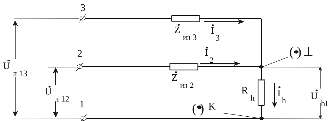
Рис. 6.11. Эквивалентная схема I варианта
