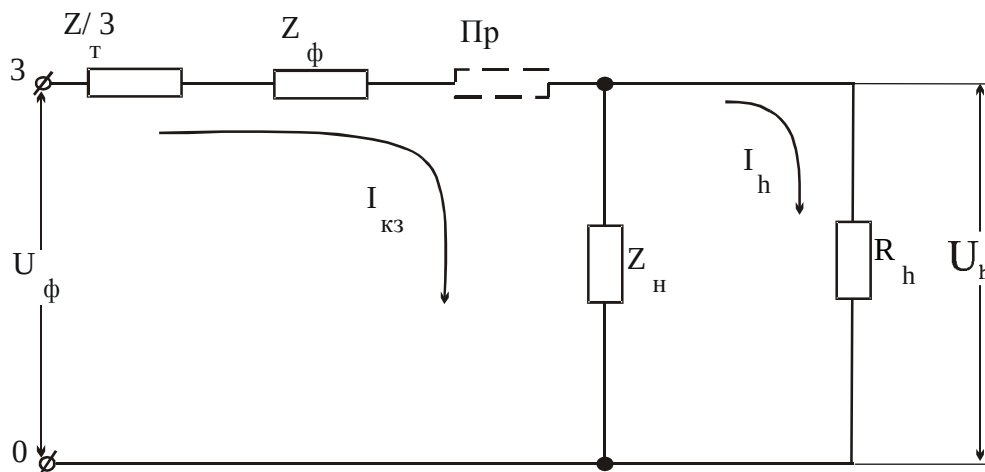
Рис. 6.15. Преобразованная эквивалентная схема зануления при отсутствии повторного заземления нулевого провода R_n
