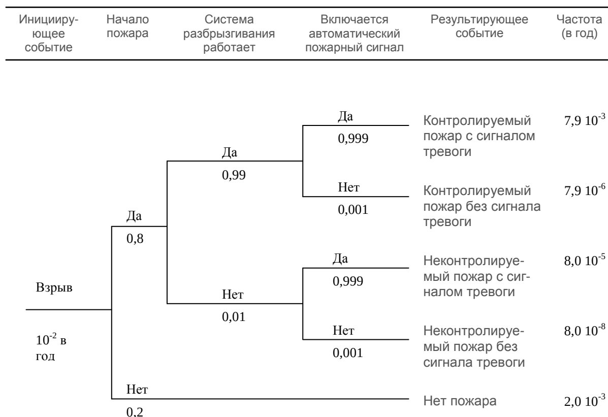
Рис. 9.1. Использование «дерева отказов» для оценки риска
