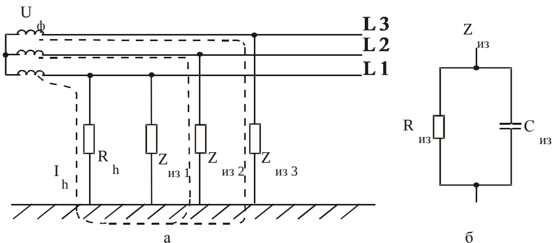
Рис. 6.5. Трехфазная сеть с изолированной нейтралью (IT) в нормальном режиме работы: а – однофазное прикосновение человека; б – сопротивление изоляции фаз относительно земли
