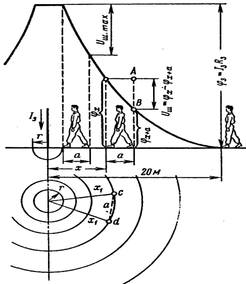
Рис. 6.3. Напряжение шага при одиночном заземлителе
