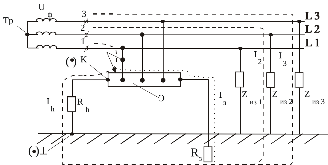
Рис. 6.10. Защитное заземление в сети с изолированной нейтралью (система IT)
