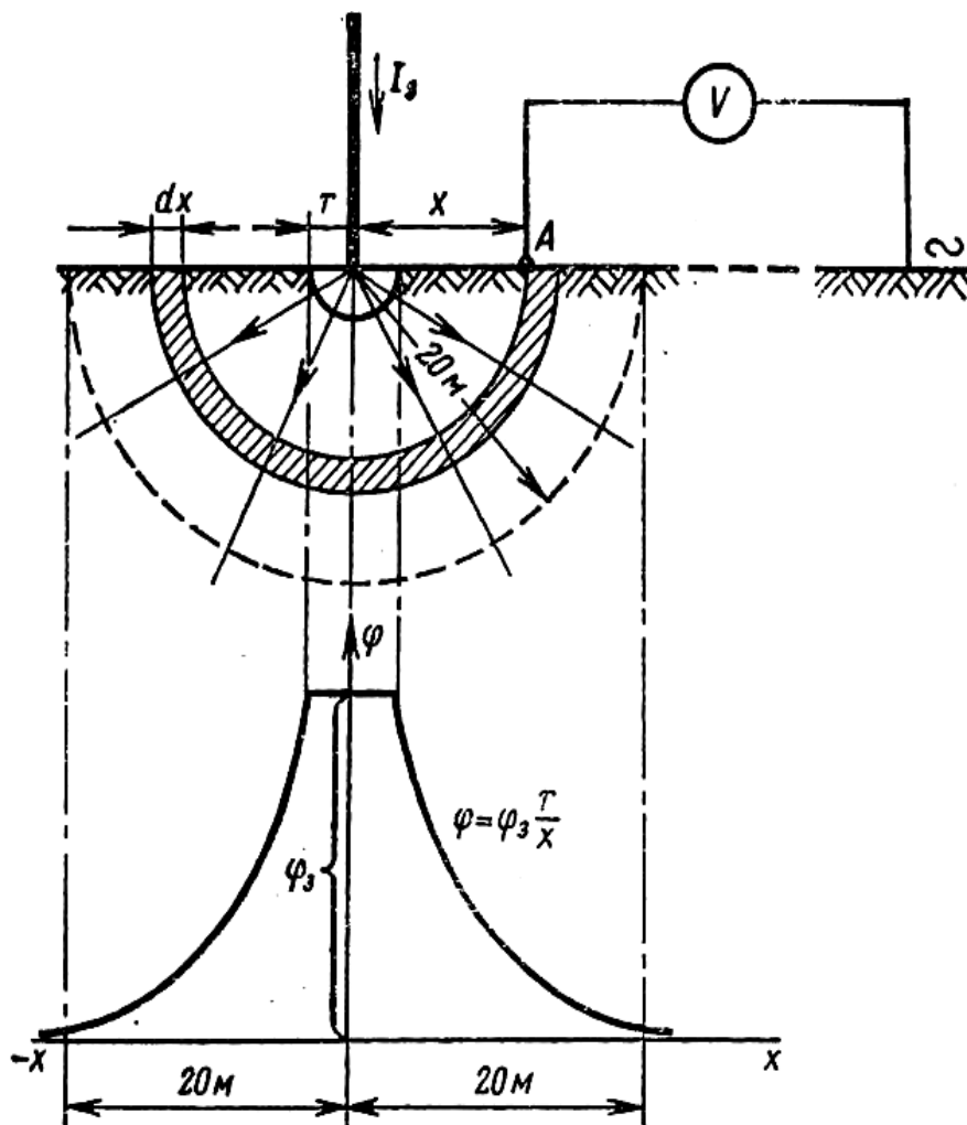
Рис. 6.1. Распределение потенциала на поверхности земли
