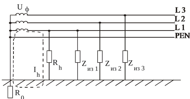
Рис. 6.7. Трехфазная сеть с глухозаземленной нейтралью (TN – C) в нормальном режиме работы
