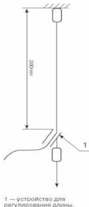
Рис.4 Испытание стропа статической нагрузкой
