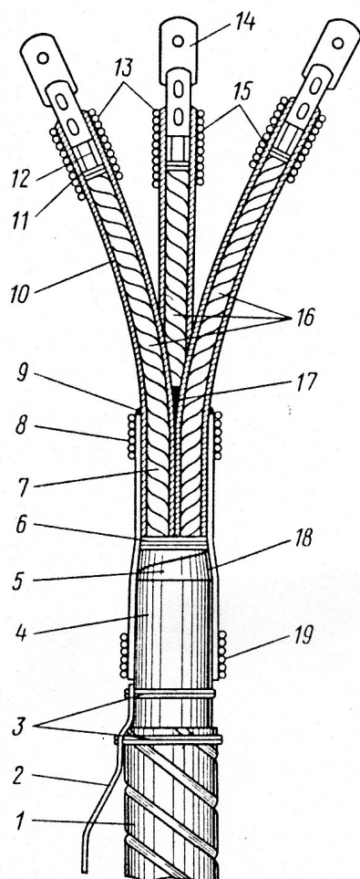
Рис. 11. Концевая заделка КВВ: 1,4 – броня и оболочка кабеля, 2 – провод заземления, 3 – проволоочные бандажы, 5 – поясная изоляция, 6,11 – бандажы из хлопчатобумажной пряжи, 7 – токопроводящая жила, 8, 15, 19 – бандажы из крученого шпата, 9 – поясная стаканообразная подмотка, 10 – подмотка жил поливинилхлоридной лентой, 12 – оголенный участок жилы, 13, 18 – выравнивающие подмотки, 14 – кабельный наконечник, 16 – участок наложения временного бандаж, 17 – наполнитель
