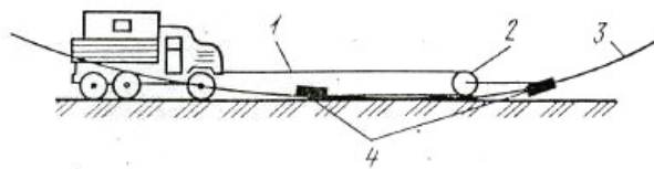
Рис. 19. Схема снятия тяжения с поврежденного провода:
