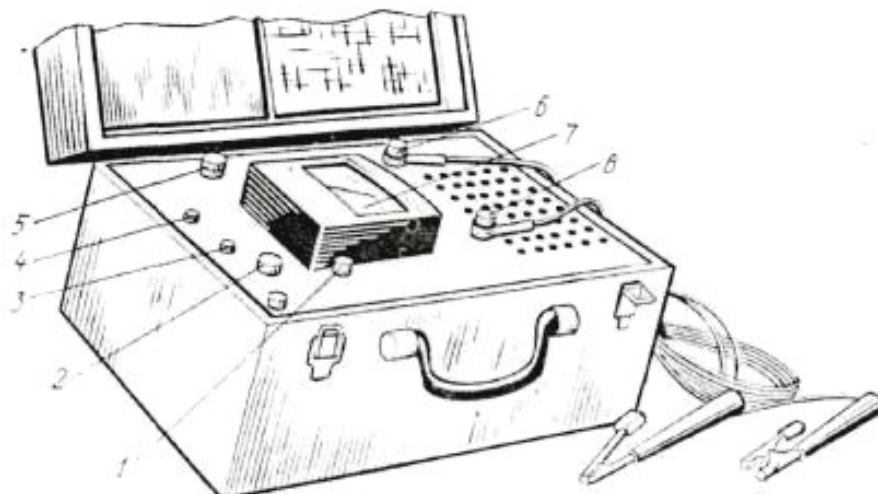
Рис. 37. Прибор М-417: 1 – лампа ( Z > 2 \text{ Ом} ); 2 – рукоятка «Калибровка»; 3 – кнопка «Проверка калибровки»; 4 – кнопка «Измерение»; 5 – лампа ( Z \neq \infty ); 6, 8 – зажимы для присоединения проводов к фазному проводу и корпусу; 7 – стрелочный прибор; 9 – пружинные соединительные зажимы
