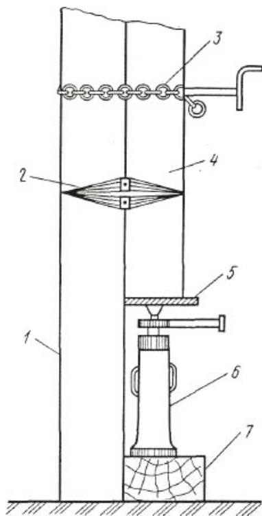
Рис. 33. Выправка опоры с помощью домкрата: 1 – приставка, 2 – проволочный бандаж, 3 – цепной бандаж, 4 – выпрямленная стойка, 5 – деревянная подкладка, 6 – винтовой домкрат, 7 – шпала
